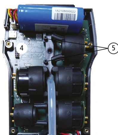
Cellule enlevée
