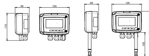
Modèle déporté
